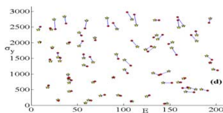
شکل 4-33: مقایسه جواب‌های دقیق و نتایج الگوریتم معکوس برای یک دسته از نتایج آزمون فرو رفتگی به دست آمده از FEA، در صفحه‌ی \sigma_y, E .
