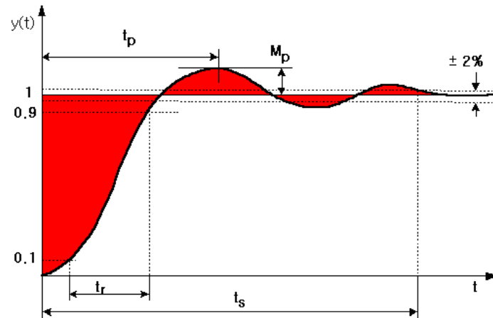
شکل 2-4: زمان صعود ( t_r )، زمان نشست ( t_s )، بیشترین فراجهش ( M_p ) و انتگرال قدر مطلق خطا (مساحت ناحیه‌ی تیره رنگ)
