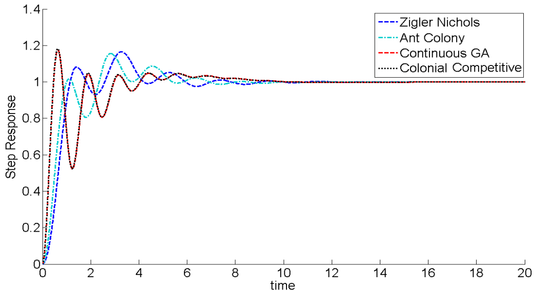
شکل 8-4: پاسخ پله‌ی سیستم به ورودی پله با استفاده از هر چهار کنترلر موجود در جدول 4-1.
