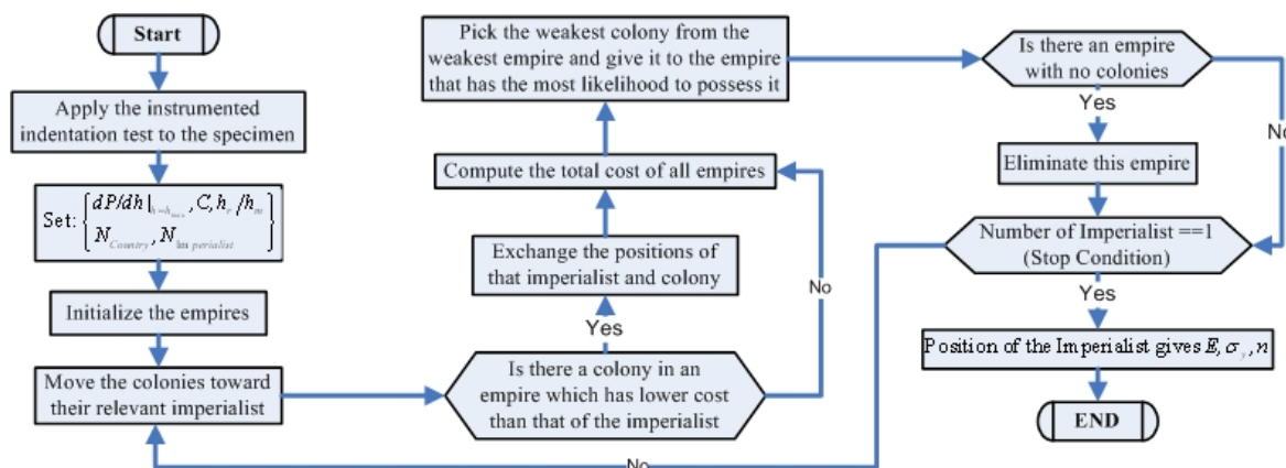
شکل 25-4: فلوچارت ICA، اعمال شده به آنالیز معکوس آزمون فرورفتگی.
