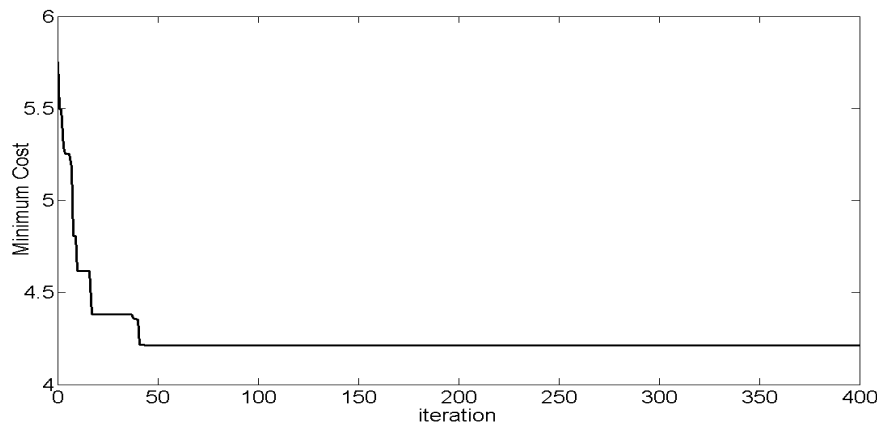
شکل 4-7: هزینه‌ی مینیمم جمعیت الگوریتم ژنتیک، بر حسب تکرار، در مسئله طراحی
