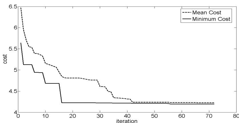
شکل 4-6: هزینه‌ی مینیمم و میانگین امپریالیست‌ها بر حسب تکرار الگوریتم، در مسئله طراحی کنترل‌کننده PID.
